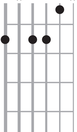
minor7b5
