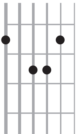
minor7
