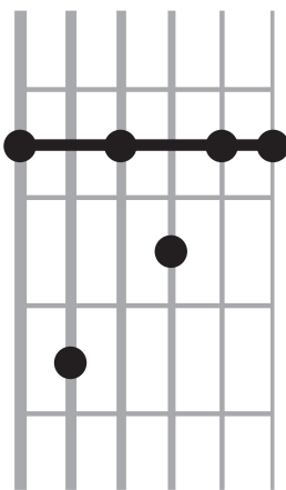
minor7b5
