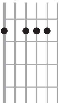
minor7
